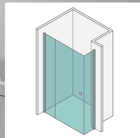
Montaż profilu do czoła ściany
